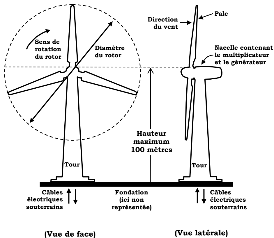
FIGURE F – SCHEMA D'ENSEMBLE D'UNE ÉOLIENNE
